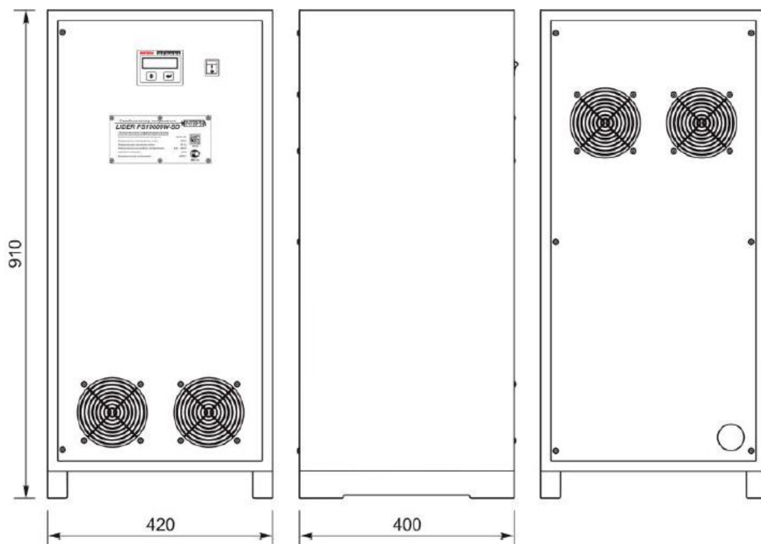
Габаритные и установочные размеры стабилизаторов напряжения переменного тока LIDER PS1000W-SD
